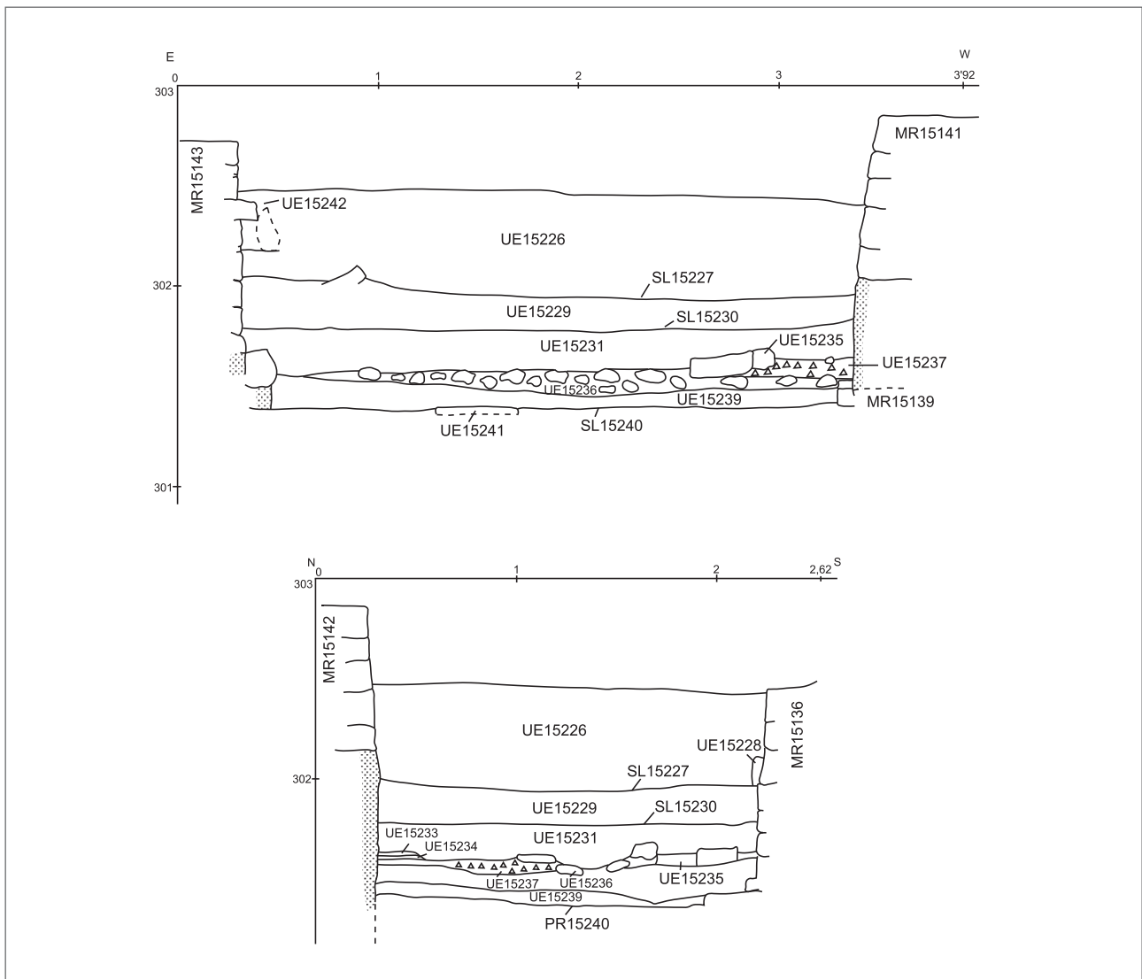
Fig. 8. Seccions sector 64
