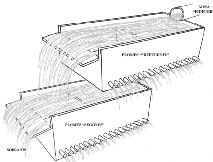
Esquema Repartidor Mina Fideuer
