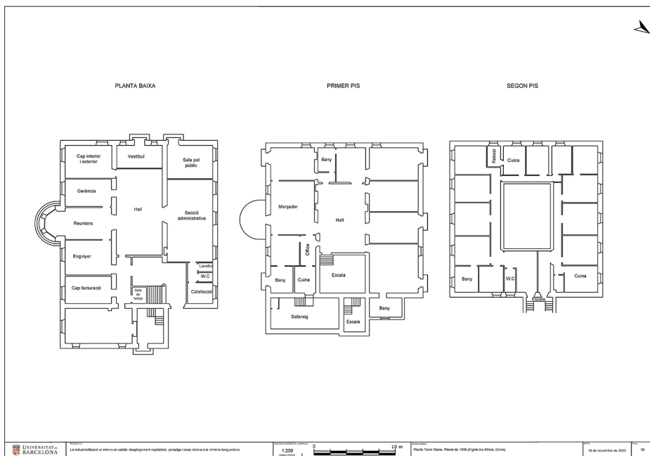
Figura 5. Planimetria de la Torre Olano (Fígols-Les Mines, Cers). Font: elaboració pròpia a partir de documents planimètrics de l'Arxiu del Museu de les Mines de Cers
