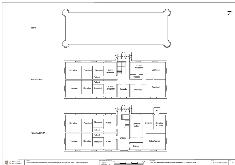
Figura 10. Planimetria de la caserna de la Guàrdia Civil original. Font: elaboració pròpia a partir de documentació planimètrica de l'Arxiu del Museu de les Mines de Cercs
