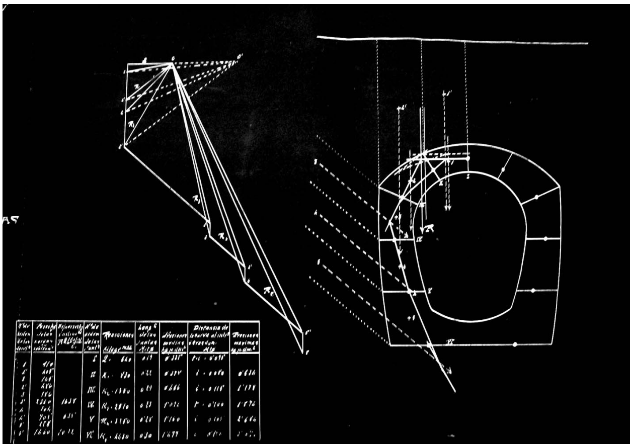
Plànol d'una secció de claveguera de l'arquitecte Pere Domènech i Roura. (AMCNM)
