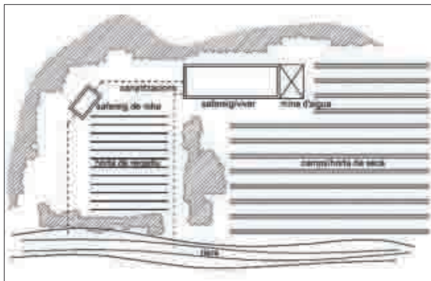
Representació esquemàtica de la situació i distribució del sistema d'aprofitament de l'aigua als horts del mas Cals de Fitor, a uns 200 metres de distància de la casa. No hi són representades les corbes de nivell, però la força emprada tradicionalment era la pròpia gravetat.
