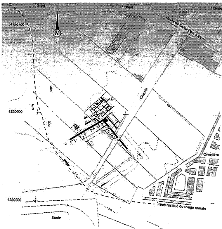
Figura 4. Plànol de la situació i estructures principals del jaciment de la Picola. Font: J. MOLINA VIDAL, «La cetaria de Picola...»
