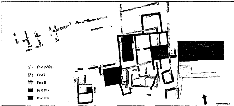
Figura 5. Fases constructives de la Picola. Font: J. MOLINA VIDAL, «La cetaria de Picola...» [Fase I: estructures d'habitació corresponents a la primera ocupació romana (finals s. I aC-principi s. II dC), fase II: estructures d'emmagatzematge (s. II-IV dC), fase III a i b: factoria de salaó (s. IV- principis del VI dC)]
