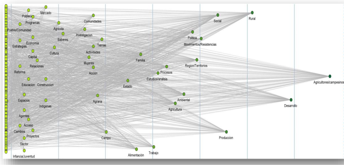
Gráfico 1. Indegree conceptual en los trabajos de Brasil presentados durante el Congreso ALASRU, 2014, México, D.F. Los conceptos con los rangos más altos son aquellos que se ubican en el extremo derecho de la gráfica. Esta visualización permitió verificar las principales preocupaciones conceptuales en los grupos de investigadores analizados (esta explicación se aplicará de aquí en adelante a todas las gráficas del presente trabajo. Fuente: Elaboración con datos de ALASRU, 2014.
