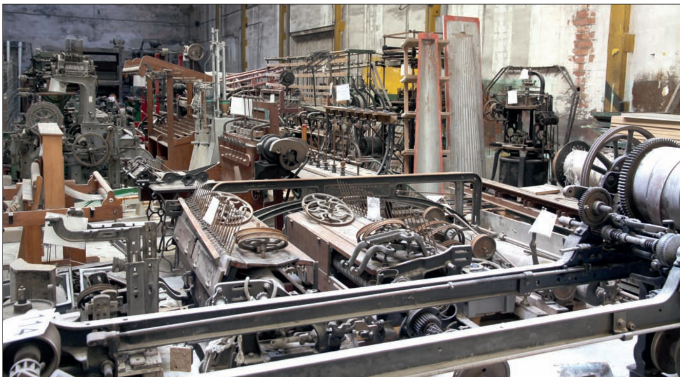
Làmina IV. Maquinària emmagatzemada actualment (2010) a la nau dels antics tallers de Hijos de Francisco Blanes.
