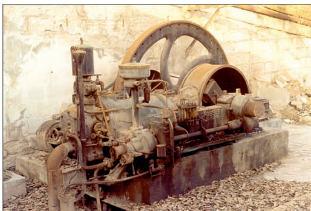
Làmina XVI. Màquina de vapor Crossley Brothers LTD (núm. 3), generador elèctric d'emergència del Teatre Calderón (Alcoi).
