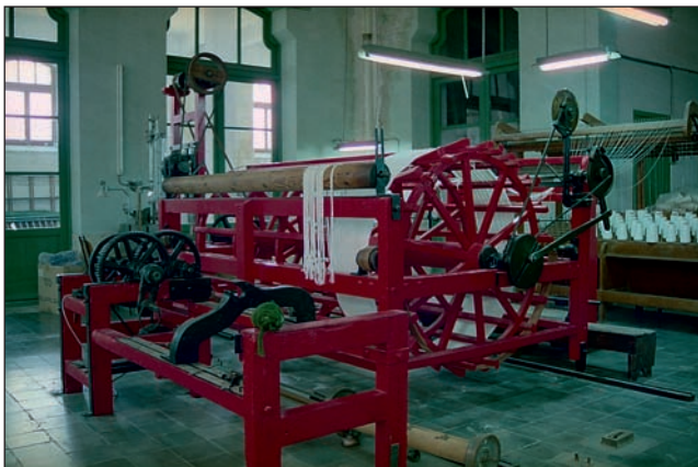
Làmina IX. Ordidor escocés (núm. 33) procedent de l'EUITIA (foto: J. M. Santacreu Soler).
