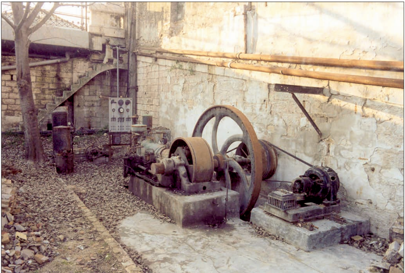
Làmina XVII. Instal·lació completa del generador elèctric d'emergència del Teatre Calderón d'Alcoi (núm. 3, 5, 7, 8 i 9)
