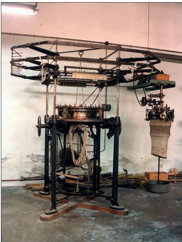
Làmina X. Teler circular de dues fontures amb cartoné (núm. 21) procedent de l'EUITIA. Ubicació original: Manufacturas Carbonell S.A. (Alcoi); (foto: J. M. Santacreu Soler).
