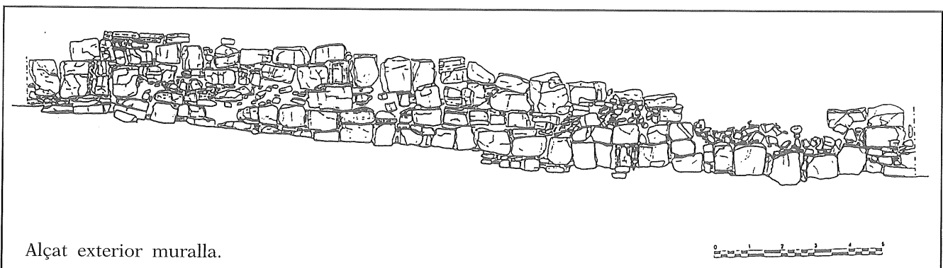
Figura 12. - Alçat exterior del parament extern de la muralla. Sector septentrional de la muralla de Torreta.
