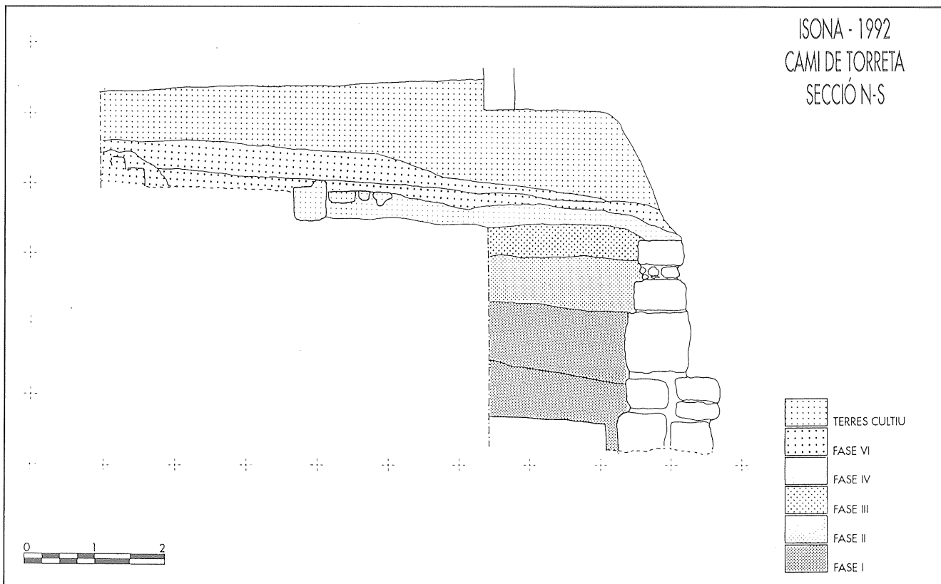
Figura 14. - Secció transversal (N-S) del sondeig intern de la muralla.
