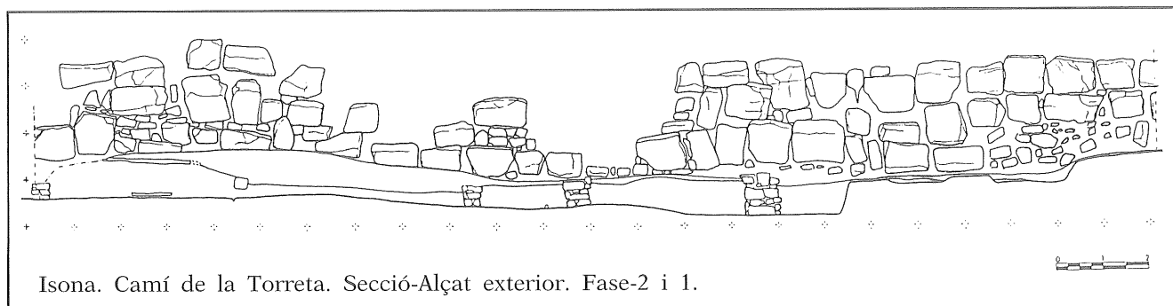
Figura 8. - Alçat exterior de la muralla. Secció de les fases -2 i -1.
