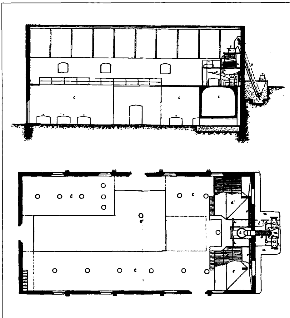
Secció longitudinal i planta del Sindicat alionenc. Fotografies publicades al llibre Cellers cooperatius de producció i venda , d'Isidre Campllonch i Romeu. Barcelona, 1917. (Autor desconegut. Data: abans de 1917)
