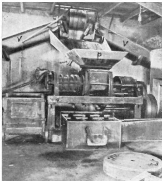
Diverses vistes de la maquinària amb què comptava el Celler. Fotografies publicades al llibre Cellers cooperatius de producció i venda , d'Isidre Campllonch i Romeu. Barcelona, 1917. (Autor desconegut. Data: abans de 1917)
