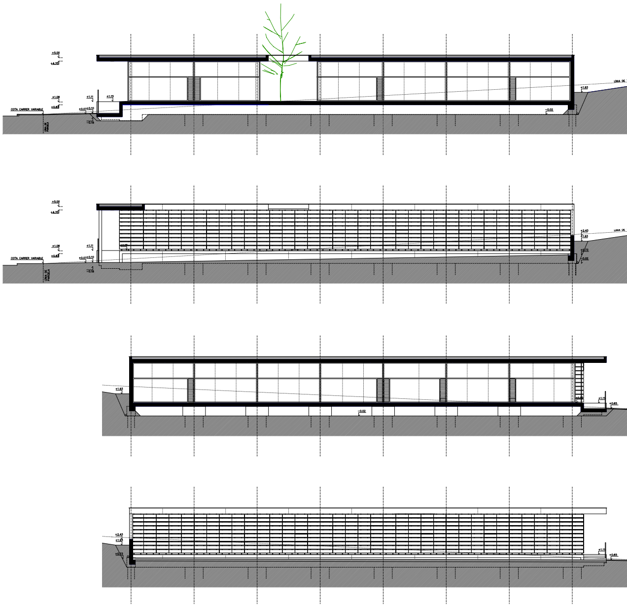
▲ Alzados y secciones
