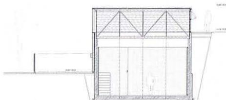
Secció · Coupe B
