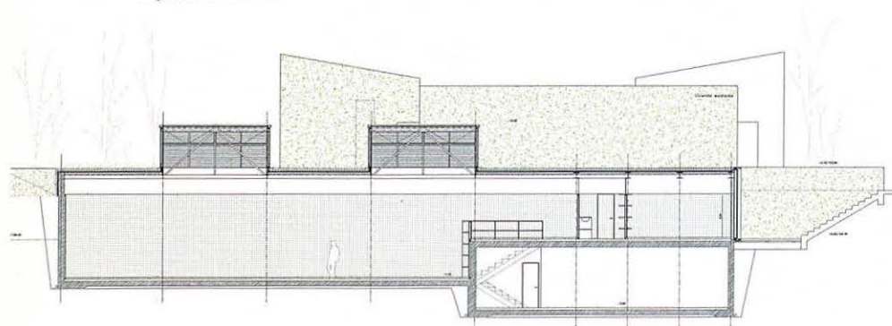
Secció · Coupe A
