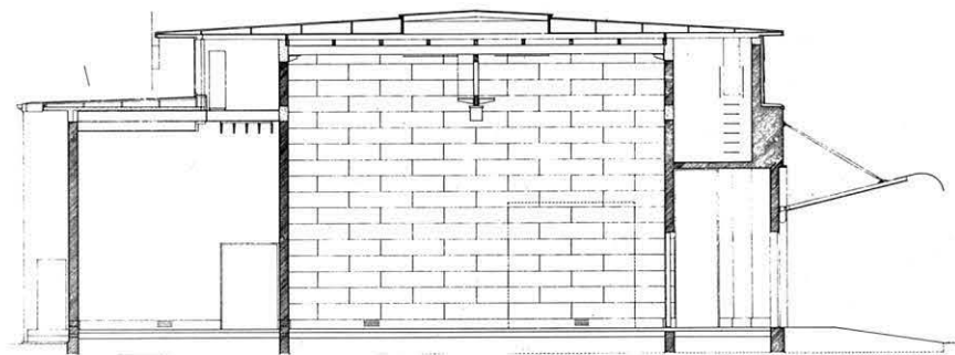
Sección.
