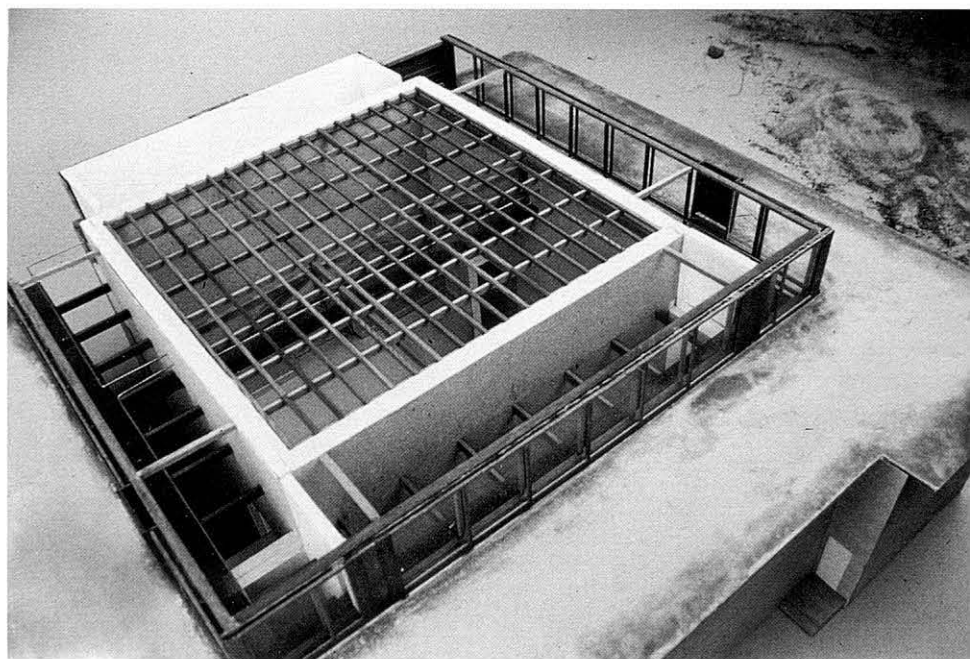
Estructura de la cubierta.
