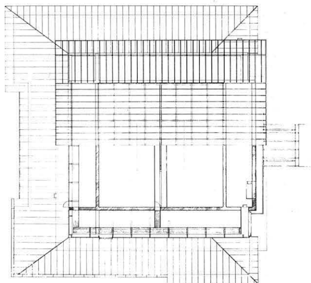
Planta lucernario y estructura de la cubierta.
