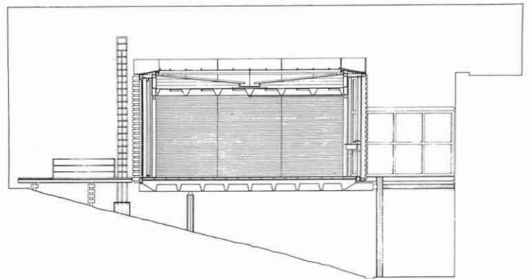
Planta i secció. Plan and section.
