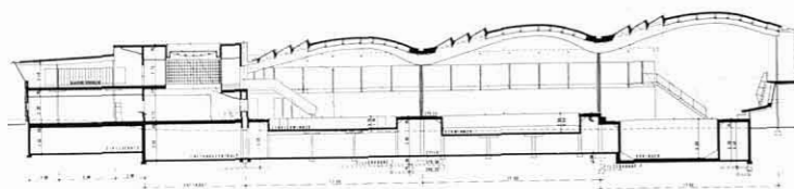
Façanes i secció del Hall de la piscina.
