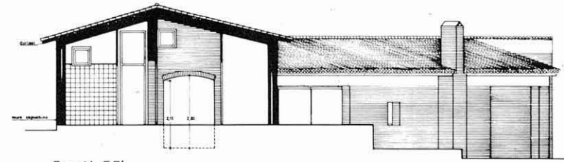
Secció CC'
