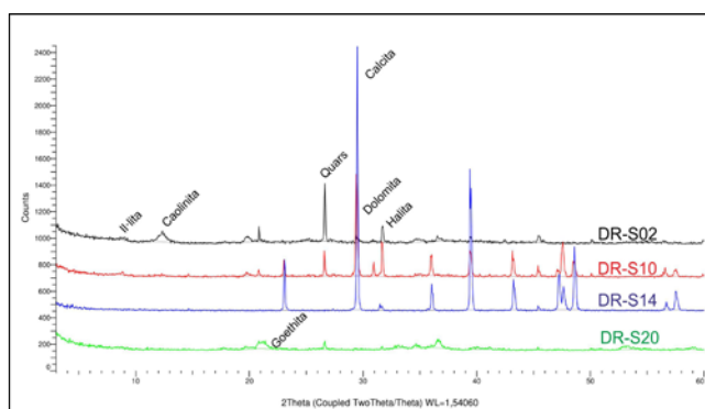
Figura 4: Difractogrames de raigs-X de mostres de sediment seleccionades.
