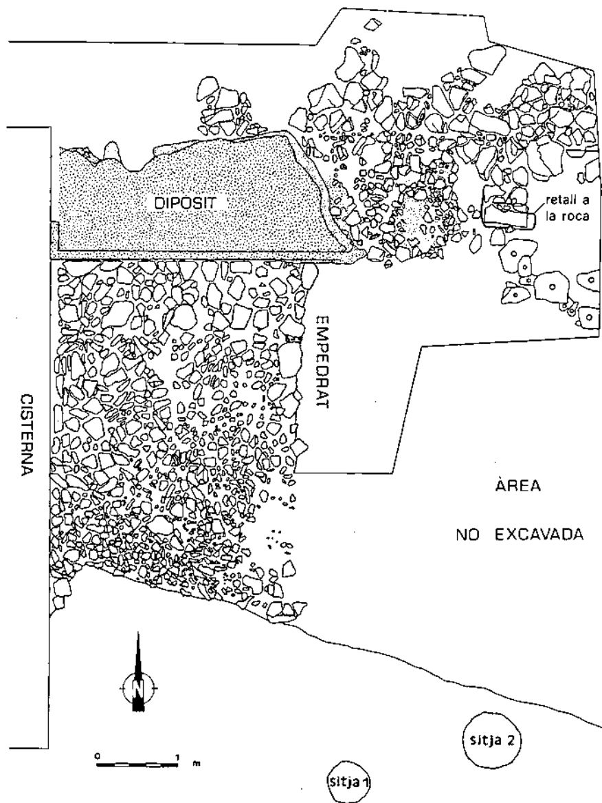
Figura 4: Planta del dipòsit i l'empedrat d'època romana adossats a la cisterna.
