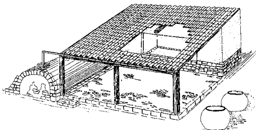
Figura 6: Reconstitució hipotètica de l'estructura romana descoberta.
