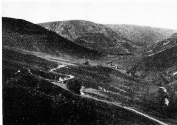
Parallel Roads de Glen Roy, Inverness-shire. (Foto Servicio Geológico de Gran Bretaña).
