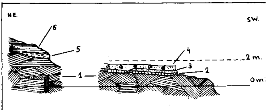
FIGURA 4. Corte del yacimiento de Carnatge (Coll d'en Rebassa). 1. Duna Rissienne cuya base se hunde en el mar. 2. Limos rojizos. 3. Costra arenosa. 4. Nivel marino Tiriense con fósiles. 5. Limos rosado-amarillentos. 6. Duna Würmiense de grano grueso.
