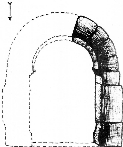
Arc de mig punt peraltat del qual se n'han recuperat quatre dovelles. (Dibuix de Joan Ramon Corts).
