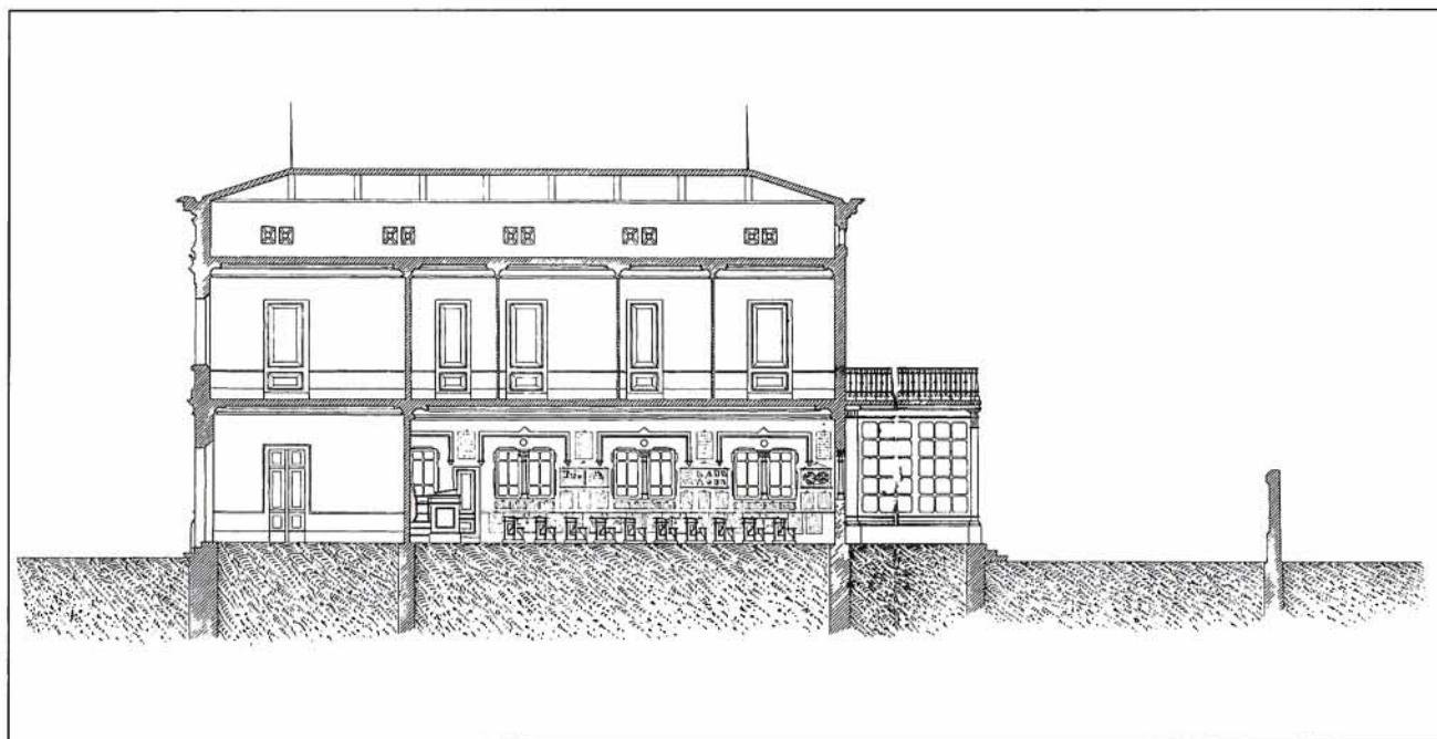
Projecte d'Escola Pública. 10 de desembre de 1885. Secció longitudinal.
