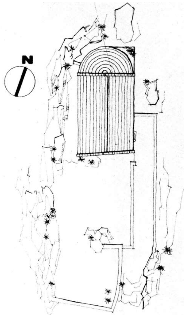
Planta de l'església i el seu entorn, que va servir a Joan Bassegoda per classificar l'església dins del grup de "muro de fachada desviado". Extret del llibre De re restauratoria , Càtedra Gaudí, UPC, 1973.
