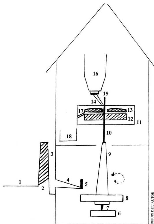
Esquema del funcionament d'un molí fariner tipus ARXIU AMBIT
