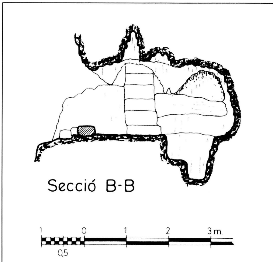
Secció transversal.
