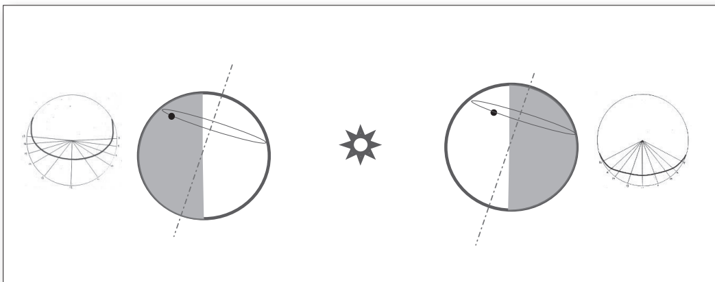
Fig. 9. Duración del día y la noche en los solsticios.
