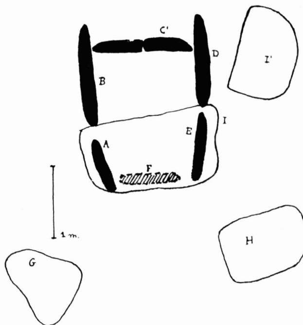
Fig. 1. — Planta del sepulcro megalítico de «Vinyes Mortes) I, Pau (Alto Ampurdán). 1 : 50.
