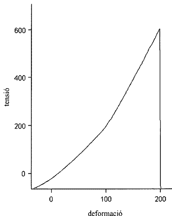
Figura 5. Gràfic tensió-deformació que representa una alta resistència mecànica a la fractura transversal ( \sigma_{max} ) d'una àmfora ibèrica.
