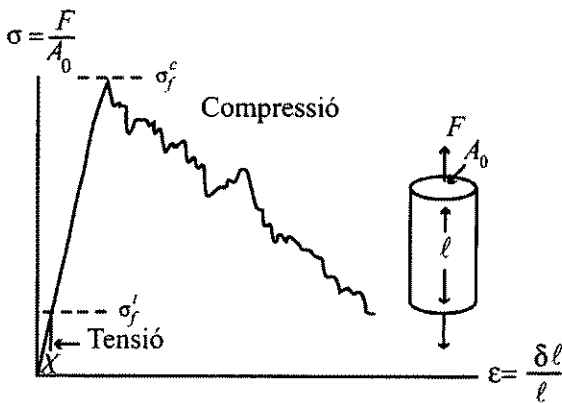
Figura 2. Gràfic resultant en aplicar una força de tensió per compressió sobre una ceràmica, on \sigma és el total de la força aplicada, \sigma_f^t és la resistència a la tensió, \sigma_f^c és la resistència a la compressió i \epsilon és la càrrega axial (Ashby 2003).
