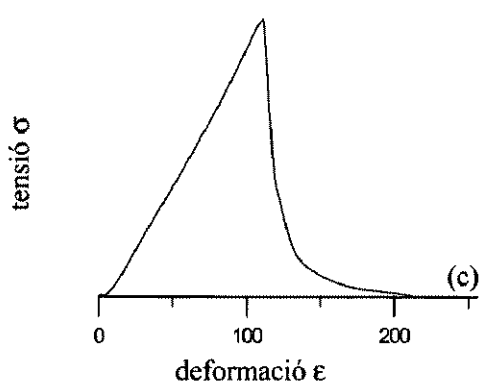
Figura 6. Gràfics tensió-deformació que representen diferents graus de resistència mecànica a la fractura ( \sigma_{max} ) de diversos contenidors d'època romana: a: resistència alta i fractura inestable; b: resistència mitjana i fractura quasi semi-estable; c: resistència baixa i fractura semi-estable.
