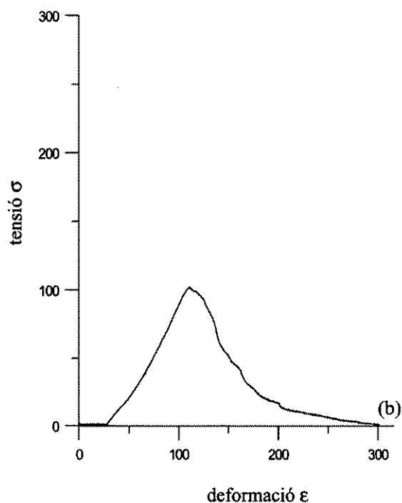
Figura 7. Gràfics tensió-deformació que representen graus diferents de tenacitat a la fractura de les àmfores d'època romana: a: Material poc tenaç, resistent a la fractura però poc resistent a la seva propagació; b: material tenaç, poc resistent a la fractura però resistent a la seva propagació.
