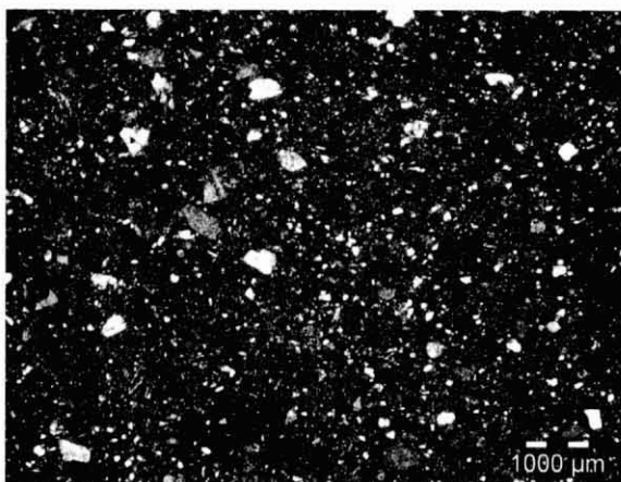
Figura 1. a: Microfotografia de la pasta ceràmica d'una àmfora ibèrica en làmina prima. Observació per microscopi petrogràfic utilitzant nicols creuats, a 40X; b: Microfotografia de la pasta ceràmica d'una àmfora romana de tonalitat vermella, procedent de Ca l'Arnau (Cabrera de Mar) de típica pasta "Tarraconense". Observació per microscopi petrogràfic utilitzant nicols creuats, a 40X; c: Microfotografia de la pasta ceràmica d'una àmfora romana procedent del Vilarenc (Calafell). Observació per microscopi petrogràfic utilitzant nicols creuats, a 40X.
