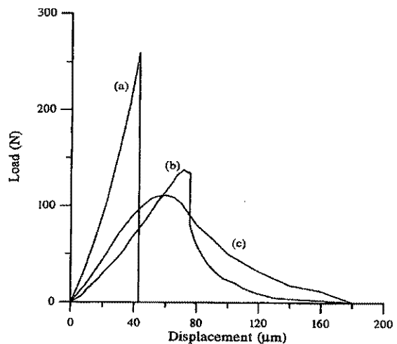
Figura 3. Gràfic força-desplaçament mostrant les corbes típiques del trencament inestable (a), semi-estable (b) i estable (c) resultants de l'aplicació d'una força (Tite/Killikoglou/Vekinis 2001).
