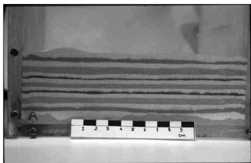
Fig. 3 – Los estratos de material más grueso no deben exceder los 2 centímetros. Los estratos finos de marcadores cinemáticos (polvo de cemento, azafrán y caril) no deben exceder los 2 milímetros. Los estratos deberán tener el aspecto más homogéneo y continuo posible. Imagen de la posición inicial, antes del inicio de la experiencia.
