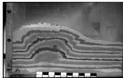
Fig. 5 – Continuando con el hinchado del globo por medio del tubo de plástico, se desarrollan cabalgamientos de alto y bajo ángulo en diversas zonas, dependiendo de la proximidad de la zona de empuje.
