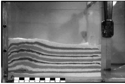
Fig. 11 – Se observa el desarrollo de pliegues con un elevado radio de curvatura en las proximidades de la intrusión y la fracturación y fallamiento en los estratos formados por polvos más finos (= estratos más resistentes). Se observa todavía el engrosamiento de algunos niveles de arenas en las secuencias sedimentarias inferiores.
