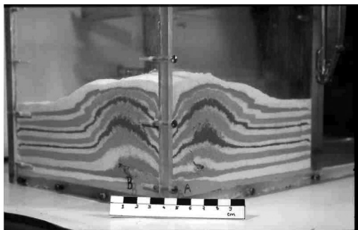
Fig. 13 – Aspecto de la experiencia observándose dos dimensiones en el espacio, secciones A y B. Vista tridimensional del módulo.
