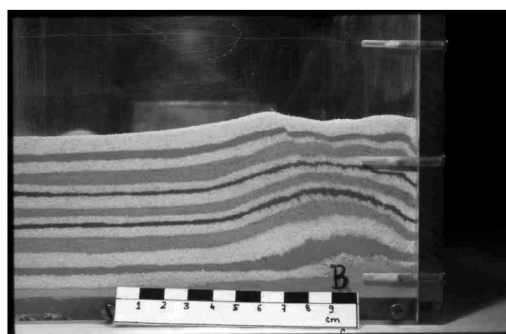
Fig. 10 – Continuación de la deformación, debida al empuje de la estructura. Nótese que mientras en la parte inferior de la caja dominan los pliegues, en la superior los estratos presentan fallas normales e inversas. Ésta es una oportunidad para introducir el concepto de piso estructural.
