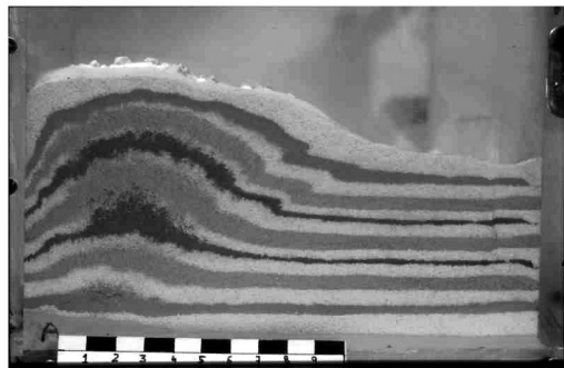
Fig. 12 – Es importante que la escala esté siempre presente para que se puedan obtener conclusiones para los trabajos de campo que se realizarán posteriormente a la fase experimental. Las dimensiones de los pliegues y problemas de escala deben ser discutidos con los alumnos. Una vez más se observan pliegues en las zonas más profundas y fallas en las zonas más superficiales del modelo.
