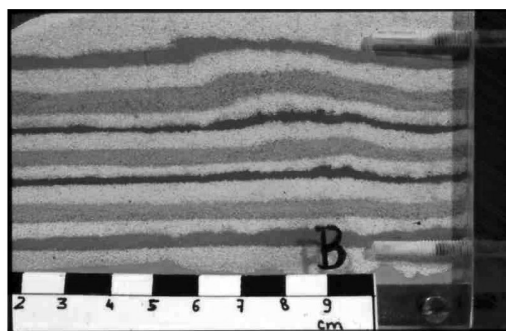
Fig. 9 – Superficie de observación B – Inicio de la deformación. Desarrollo de las primeras estructuras propias de deformación frágil, precursoras de la formación de la fallas posteriores. Desarrollo de un semi-horst, debido al comienzo del empuje hacia arriba. Las fallas desarrolladas en la zona inferior de la secuencia se propagan hacia la zona más elevada de los estratos.
