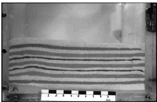
Fig. 8 – Esta figura y las siguientes muestran el segundo grupo de experimentos realizados, considerando las dos superficies de la caja (sup. A y B). Inicio de la experiencia con los estratos continuos y horizontales.
