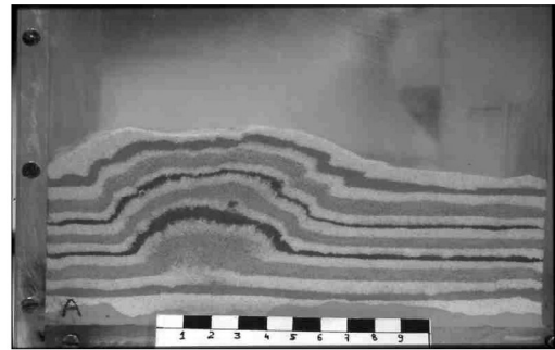
Fig. 4 – Primeros incrementos de aire en el globo. Desarrollo de pequeñas estructuras cabalgantes en la periferia de la zona de interferencia del globo. Simultáneamente tiene lugar el desarrollo de fallas normales (estructuras en graben), en la parte más elevada de la estructura como resultado del inicio del empuje (plegamiento de gran amplitud). Al continuar el hinchado del globo, las estructuras anteriores aumentan sus radios de curvatura, con el consiguiente aumento de la magnitud de los pliegues. De igual modo aumenta el desplazamiento a lo largo de las “fallas”, desarrolladas anteriormente. Nótese que los marcadores cinemáticos (polvos más finos) son extremadamente importantes en la cuantificación del movimiento, de la deformación y desarrollo de las estructuras frágiles (fallas).
