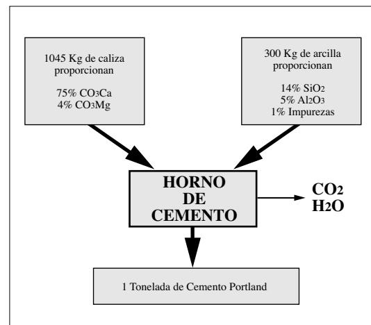
Figura 1. Materias primas necesarias para obtener una tonelada de cemento portland (según Skinner (1974), en Agueda et al., 1983).
