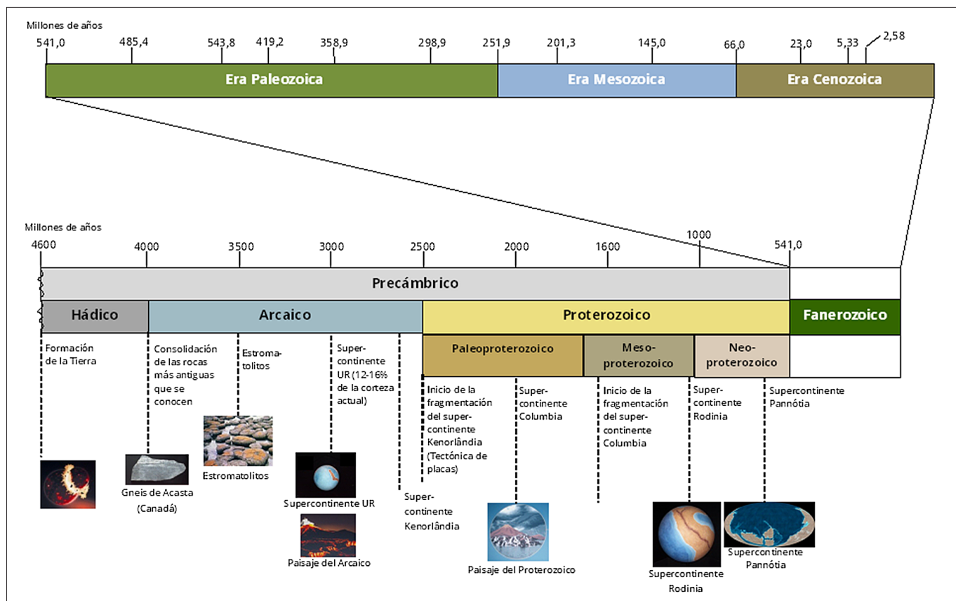
Fig. 2. Escala de tiempo geológico. Elaboración: autores.
