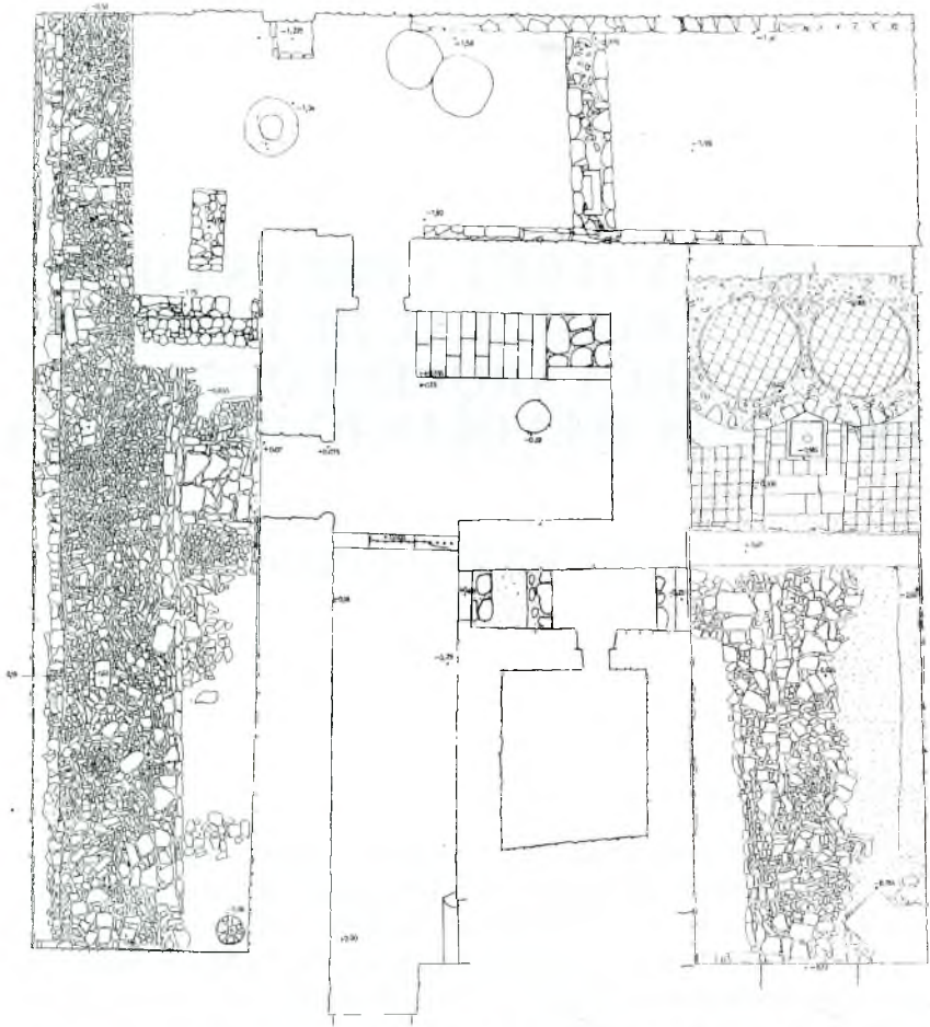
Fig. 1.- Plànol general de la planta baixa del castell, amb indicació de les principals estructures descobertes durant la intervenció.
