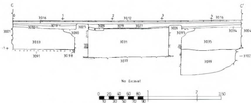
Fig. 9.- Secció estatigràfica C - C'.
