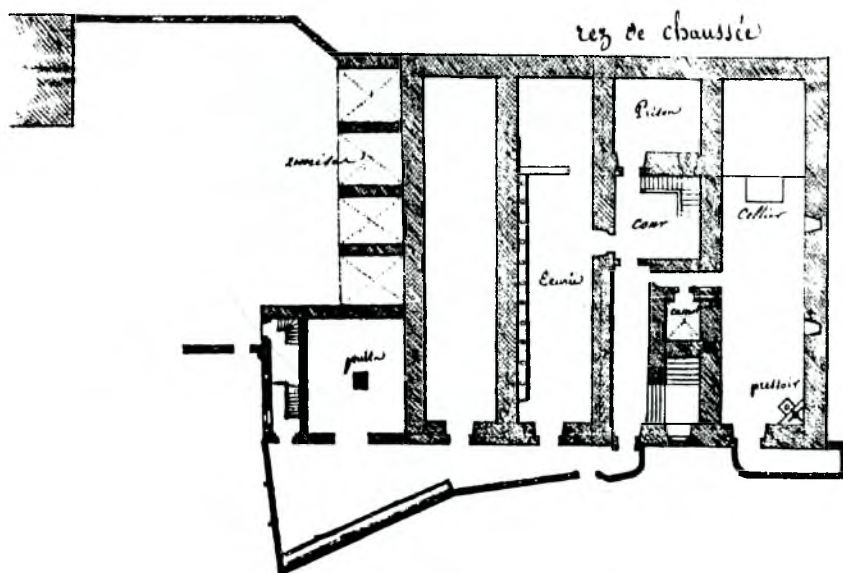
Fig. 21.- Planta general de la planta baixa del castell i defenses exteriors, segons Daigremont. Any 1823.
