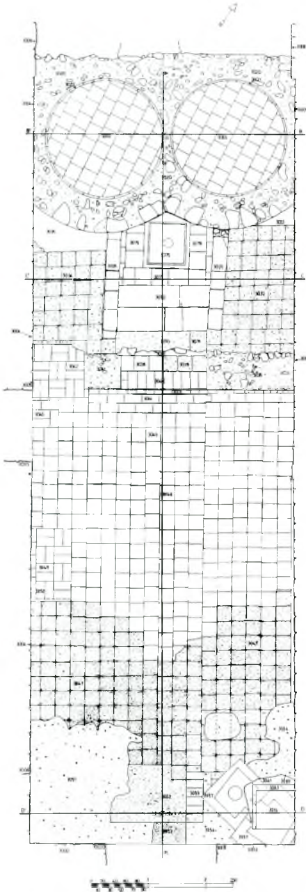
Fig. 3.- Planta general de la sala 3. Premsa de vi.
