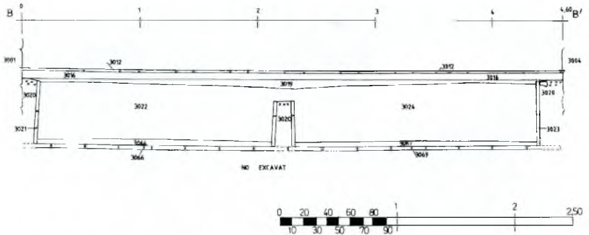
Fig. 5.- Secció estratigràfica B-B'
