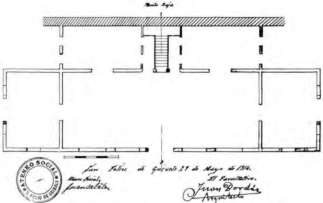
Planta de la sala-cafè que fou inaugurada el 1915. Dibuix de Joan Bordàs.
