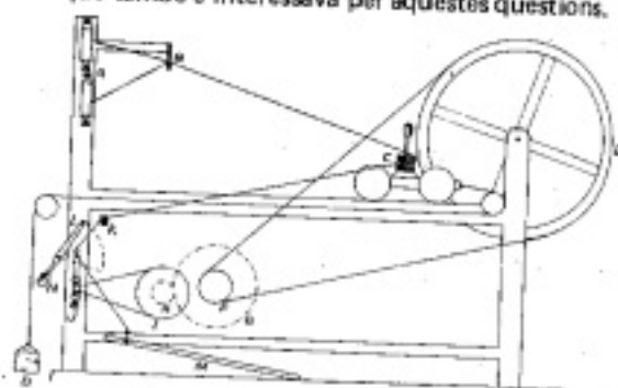
Esquema de la màquina bergadana.
