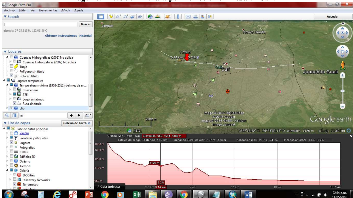
Imagen 6. Áreas de Amenaza por Remoción en Masa en Cali.
