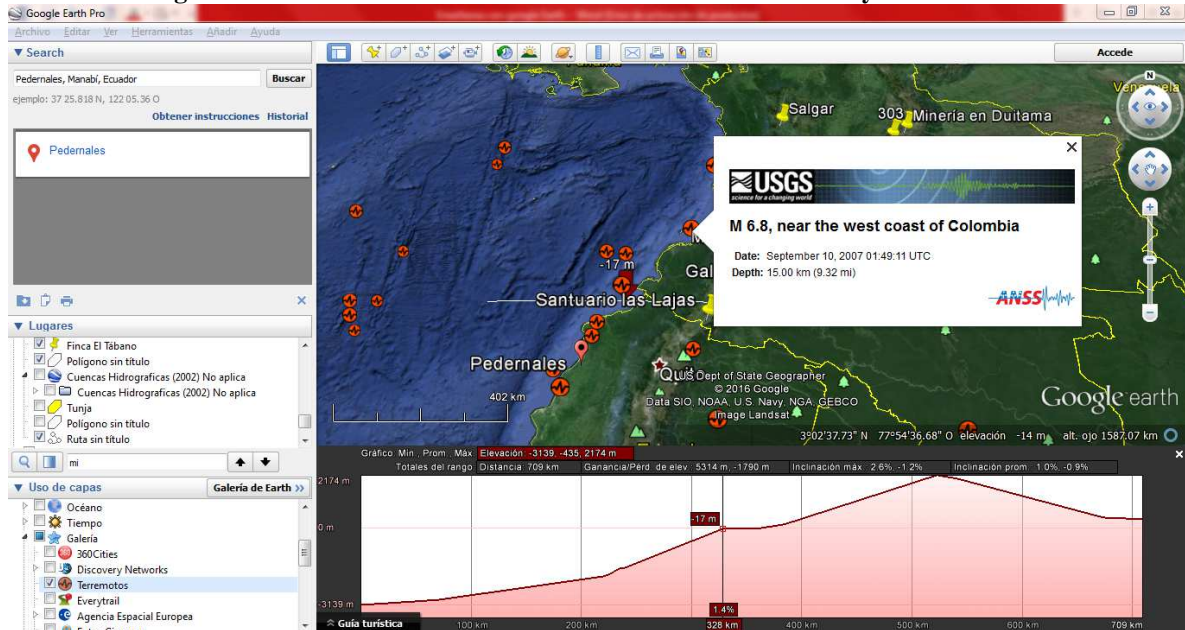
Imagen 7. Distribución de los terremotos en la costa colombiana y ecuatoriana.
