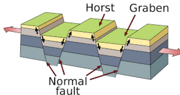
Imagen 3. Graben y Horst
