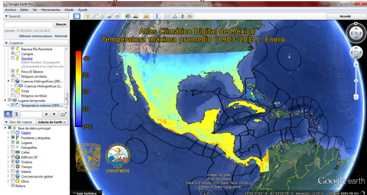
Imagen 5. Atlas Climático Digital de México.
