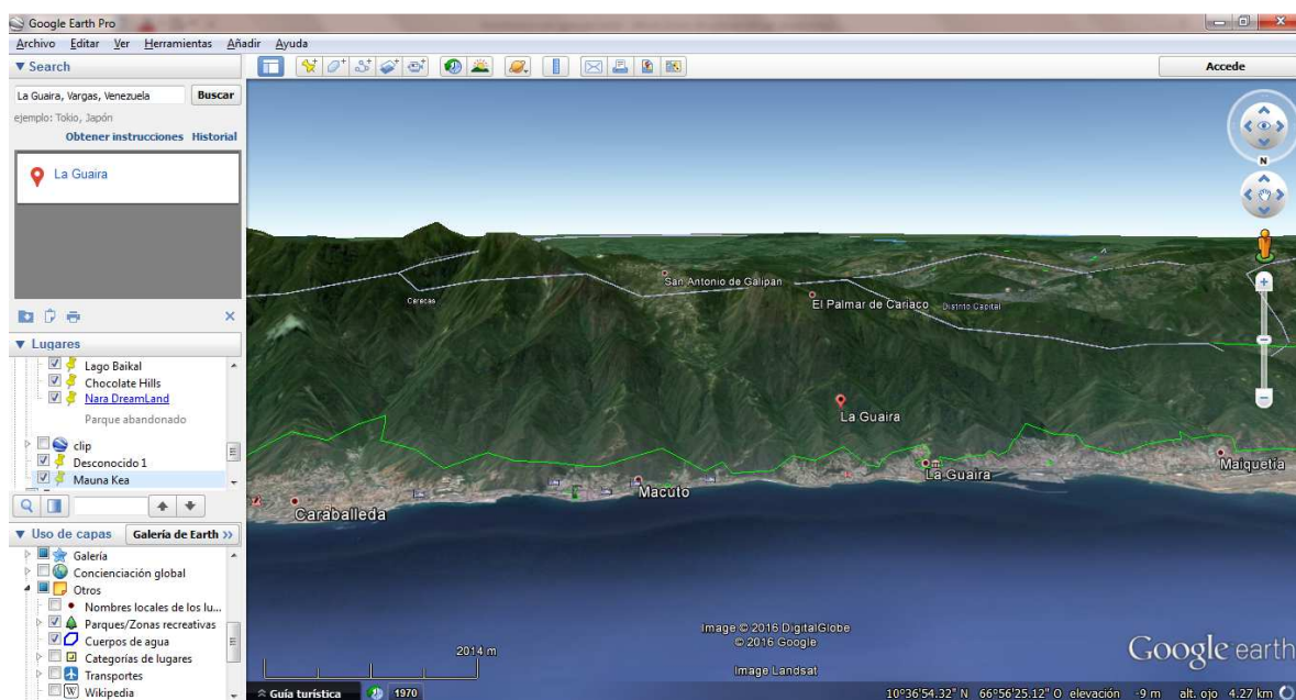
Imagen 10. Costa Atlántica venezolana, Estado de Vargas.
