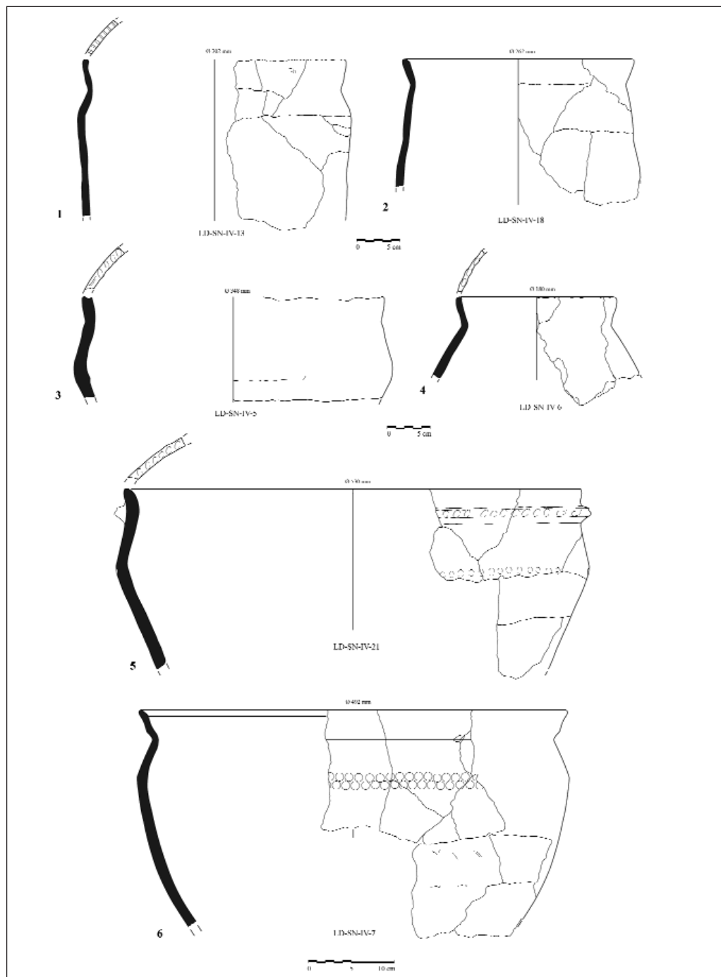
Fig. 2. Artefactes ceràmics analitzats procedents del nivell IV del sector N del fossat de la Dou.
