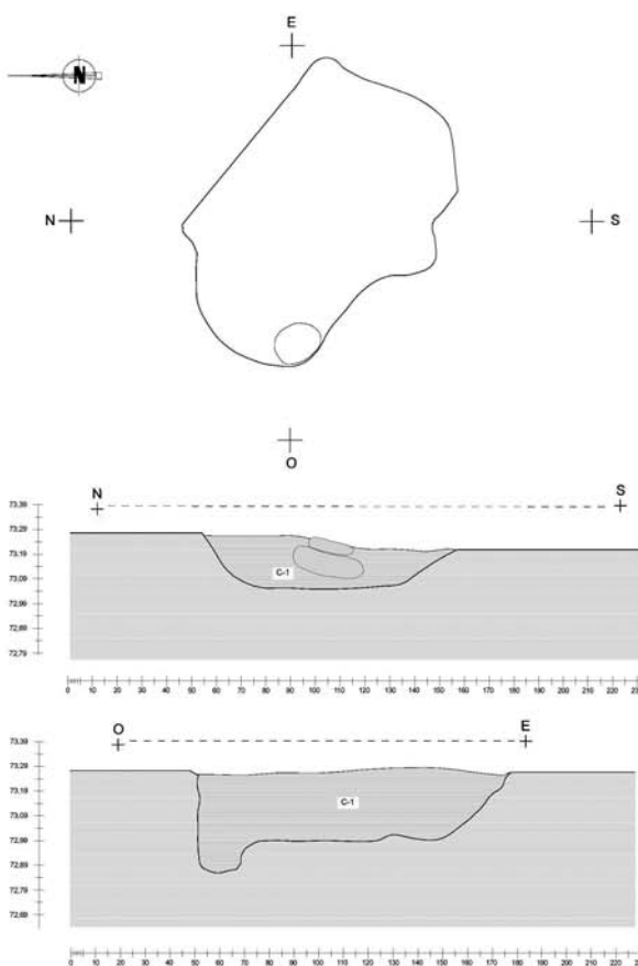
Figura 6. Planta i secció de l'estructura 52 de la Serra del Mas Bonet. Escala 1:20.
