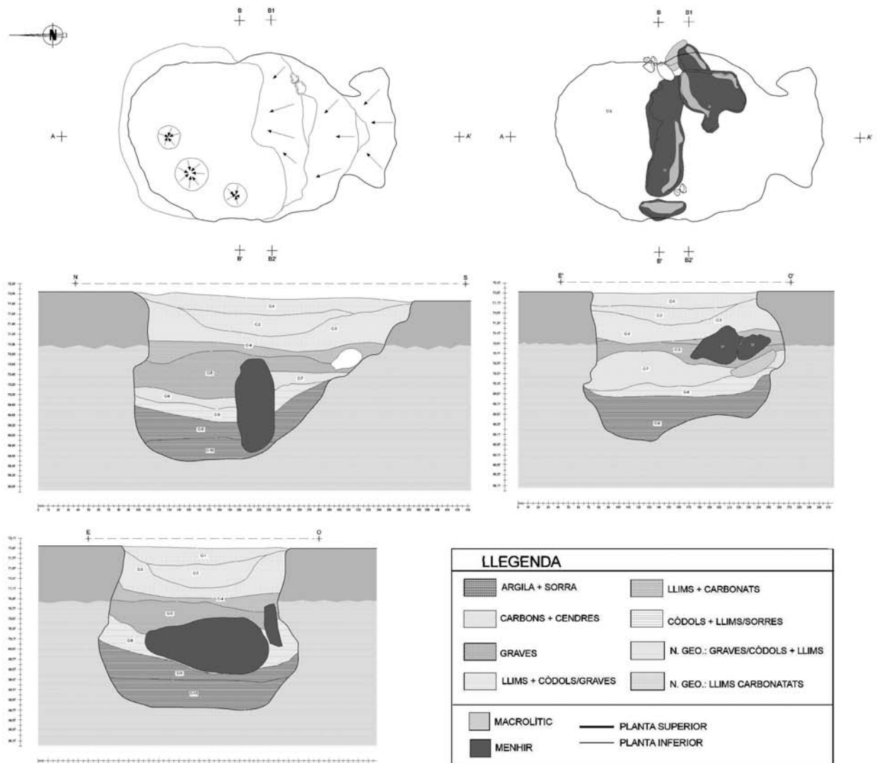
Figura 5. Planta i secció de l'estructura 17 de la Serra del Mas Bonet. Escala 1:30.
