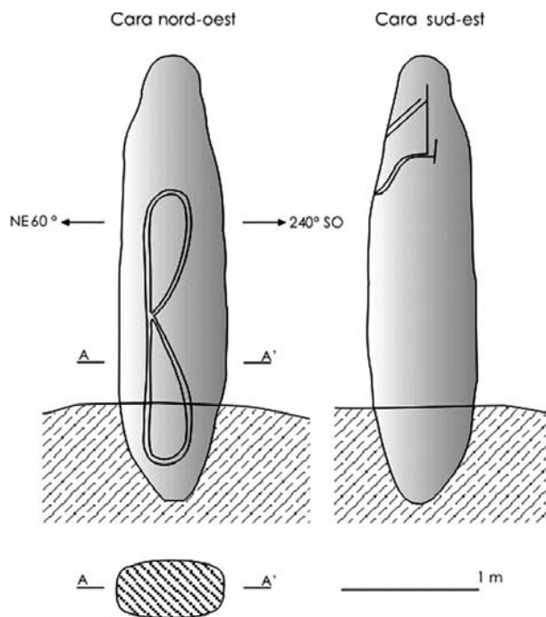
Figura 8. Calc del Gesearit dels gravats del menhir dels Palaua (Agullana, Alt Empordà), 1987 .
