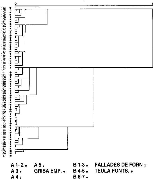
Fig. 35.- Dendograma jerarquitzat a partir de les dades aportades per les anàlisis químico-quantitatives realitzades per fluorescència de raigs X.
