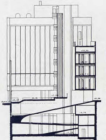
sección r-r
