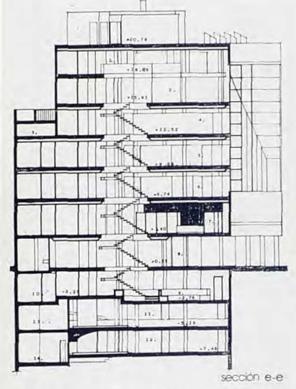
sección e-e
