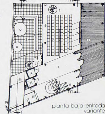
planta baja-entrada
