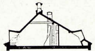
Sección
