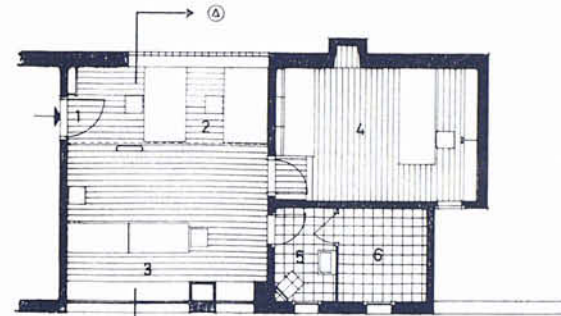
PLANTA ESTUDIO
