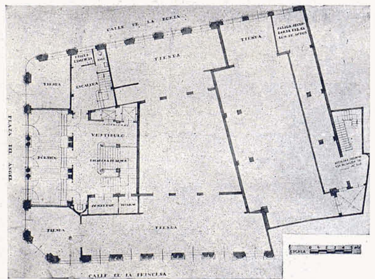
Planta baja
