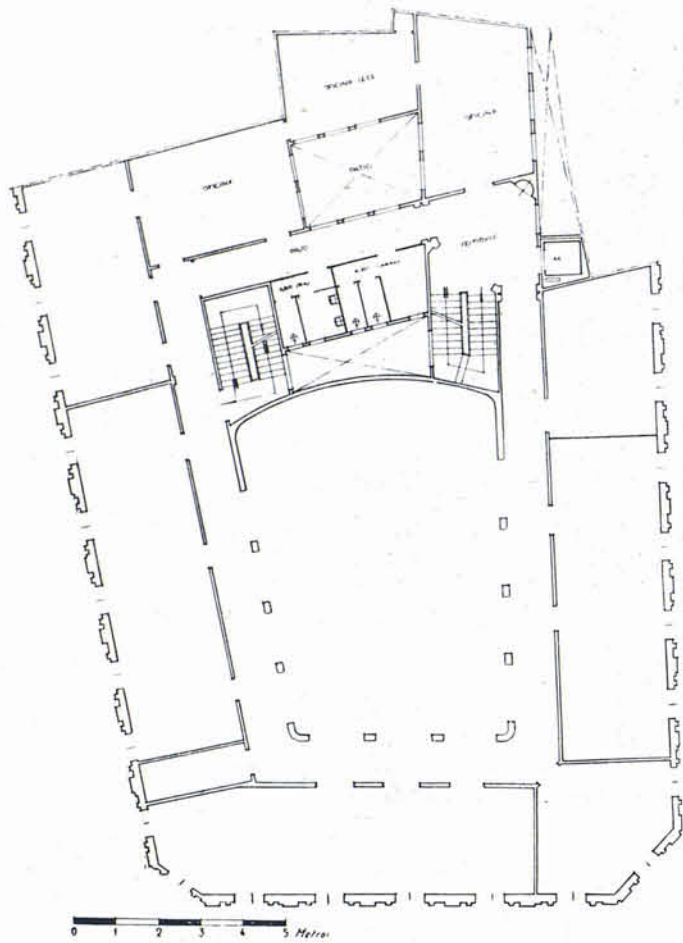
Planta principal
