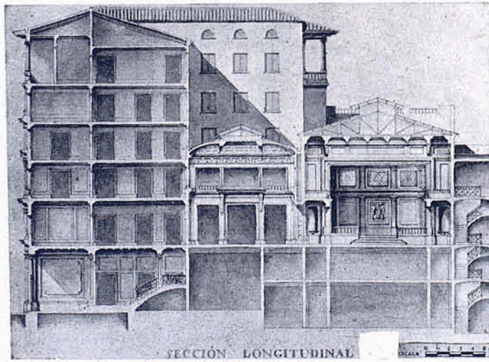
Sección longitudinal
