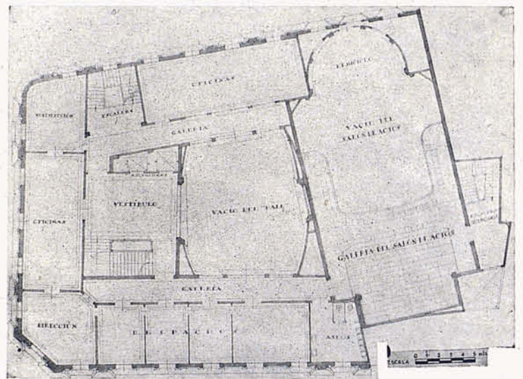
Planta piso principal
