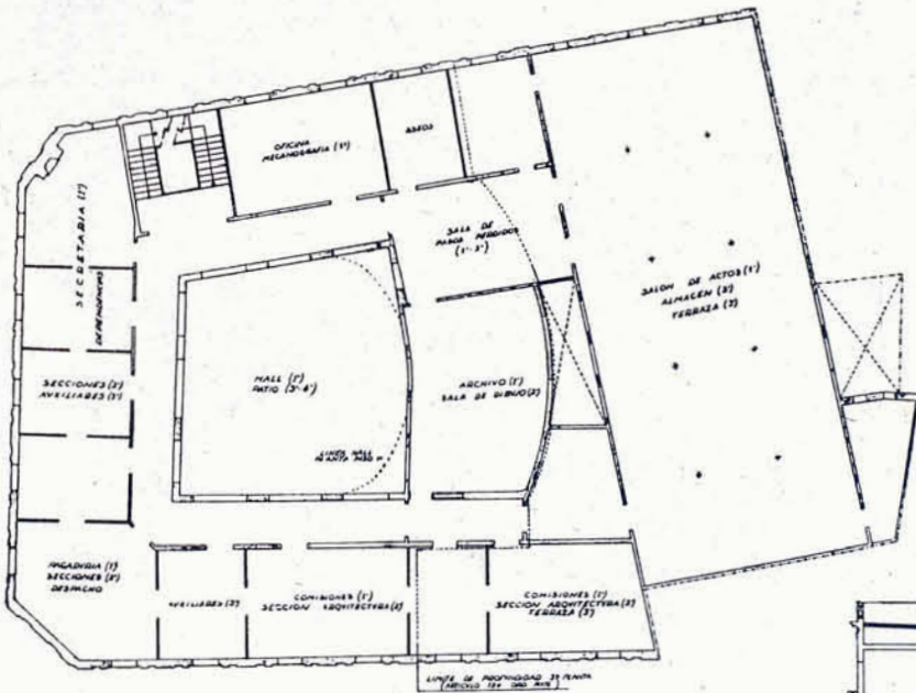
Planta pisos
