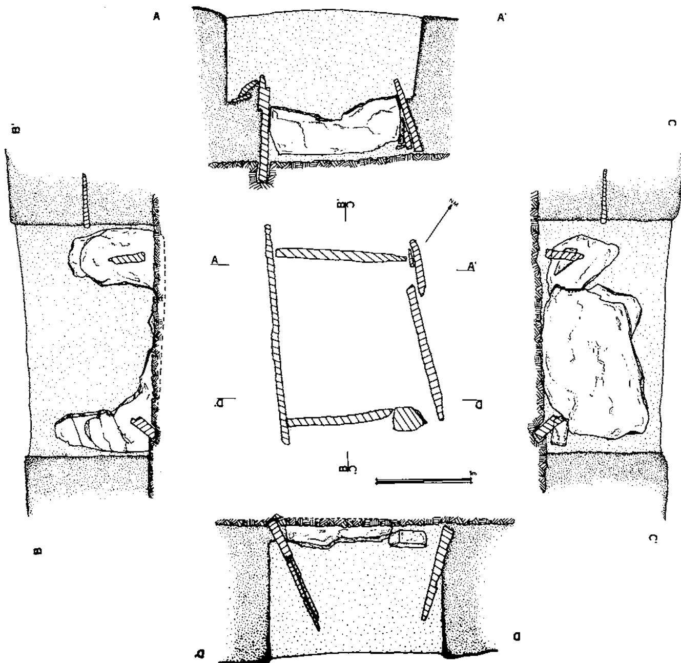
Fig. 4. Planta i alçats de la cambra de Font de la Vena.
