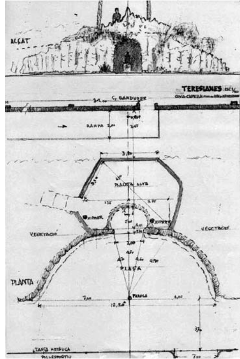
Fig. 10. Planta i alçat de la cova-capella de la M. de Déu de Montserrat. Dibuix de l'autor.
