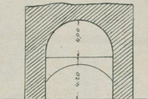
SECCIÒ CD
