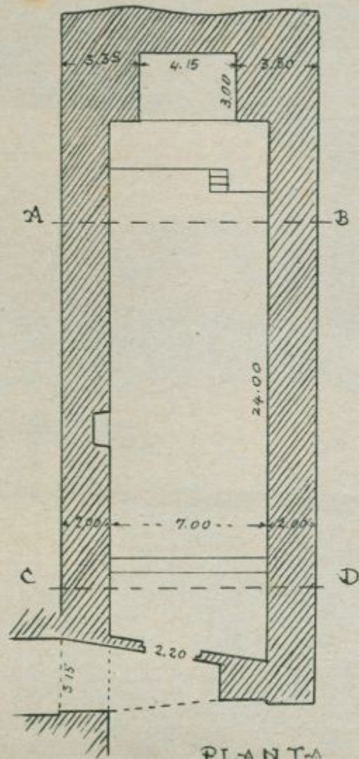
PLANTA
