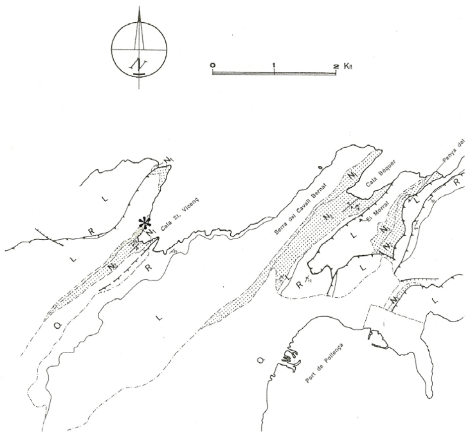
Fig. 2. Mapa geològic del sector amb la localització del jaciment estudiat: R, Triàsic superior (Retià); L, Liàsic; N1, Fm. Calcarenites de St. Elm (Aquitanià – Burdigalià inferior) on s'ubica el jaciment estudiat; N2, Fm. Turbidites de Banyalbufar (Burdigalià superior – Languià); Q, Quaternari (Modificat a partir de Gelabert et al. , 1991).
