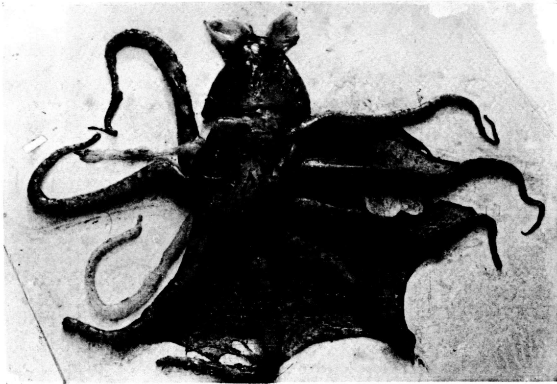
Histioteuthis bonnelli (Fér.) de aguas mallorquinas.
