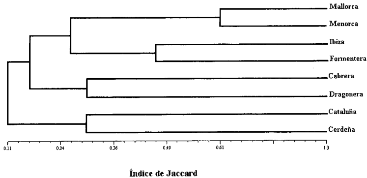
Fig. 4. Comparació de les Faunes de Chrysomelidae entre les Illes Balears, Catalunya i Sardenya usant l'índex de Jaccard.
