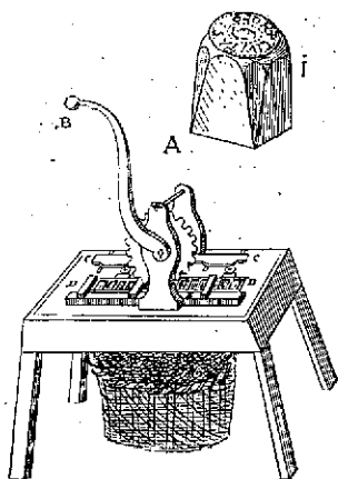
Màquina d'acordonar
