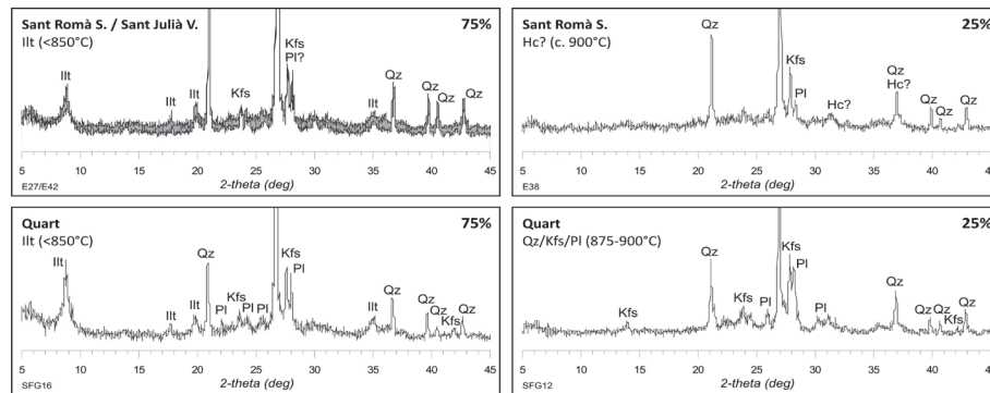
Figura 7. Temperatures de cocció estimades per DRX en ceràmica grisa medieval osonenca i gironina. Difractogrames de mostres atribuïbles a Sant Romà de Sau, Sant Julià de Vilatorrada i Quart en època medieval. El percentatge de mostres identificades de cada grup figura a la cantonada superior dreta de cada gràfic. Es pot observar com la tendència majoritària recau sobre les coccions a una temperatura inferior als 850^{\circ}\text{C} .
