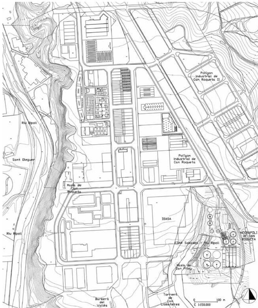
Figura 1. Emplaçament de la necròpoli amb relació al polígon industrial de Can Roqueta i a l'EDAR Sabadell-Riu Ripoll. Escala original 1:150.000. Elaboració: Xavier Carlús Martín.
